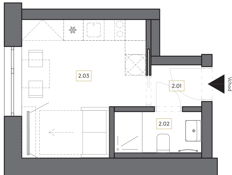
Půdorys bytu 2
