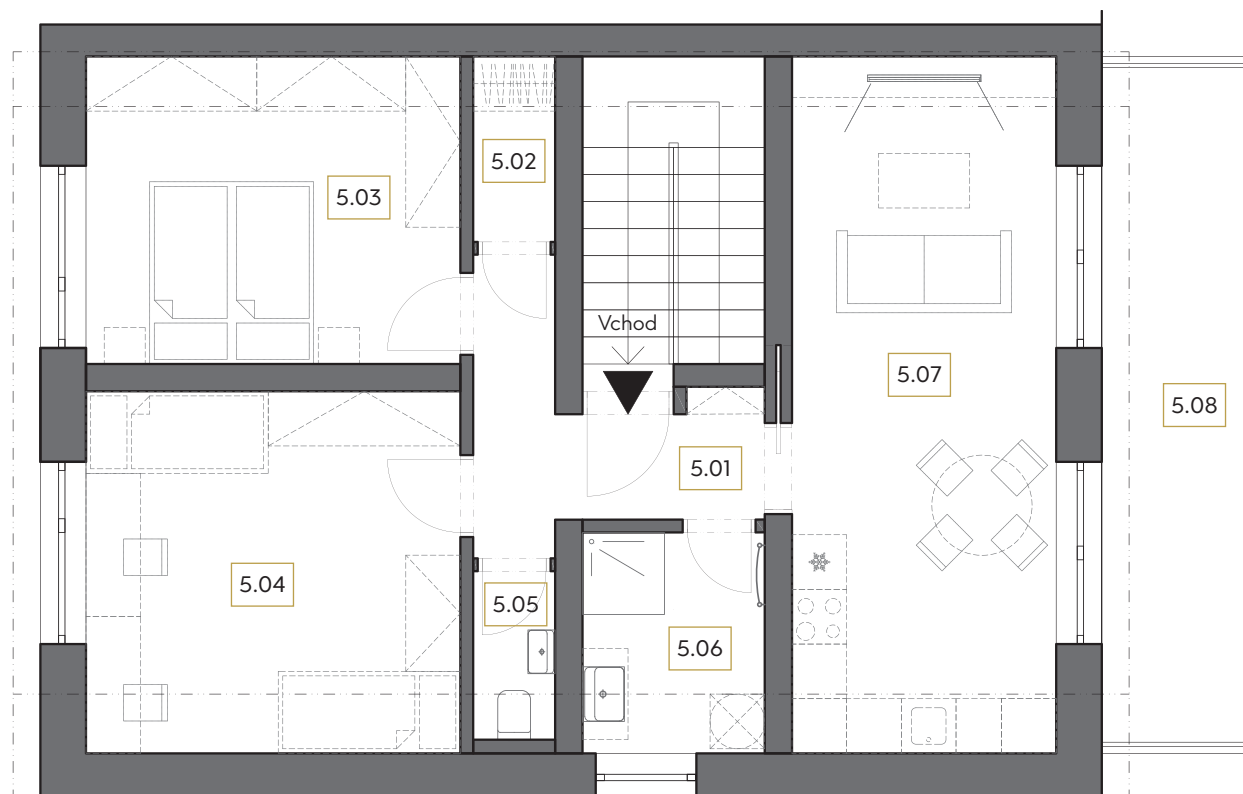
Půdorys bytu 5
