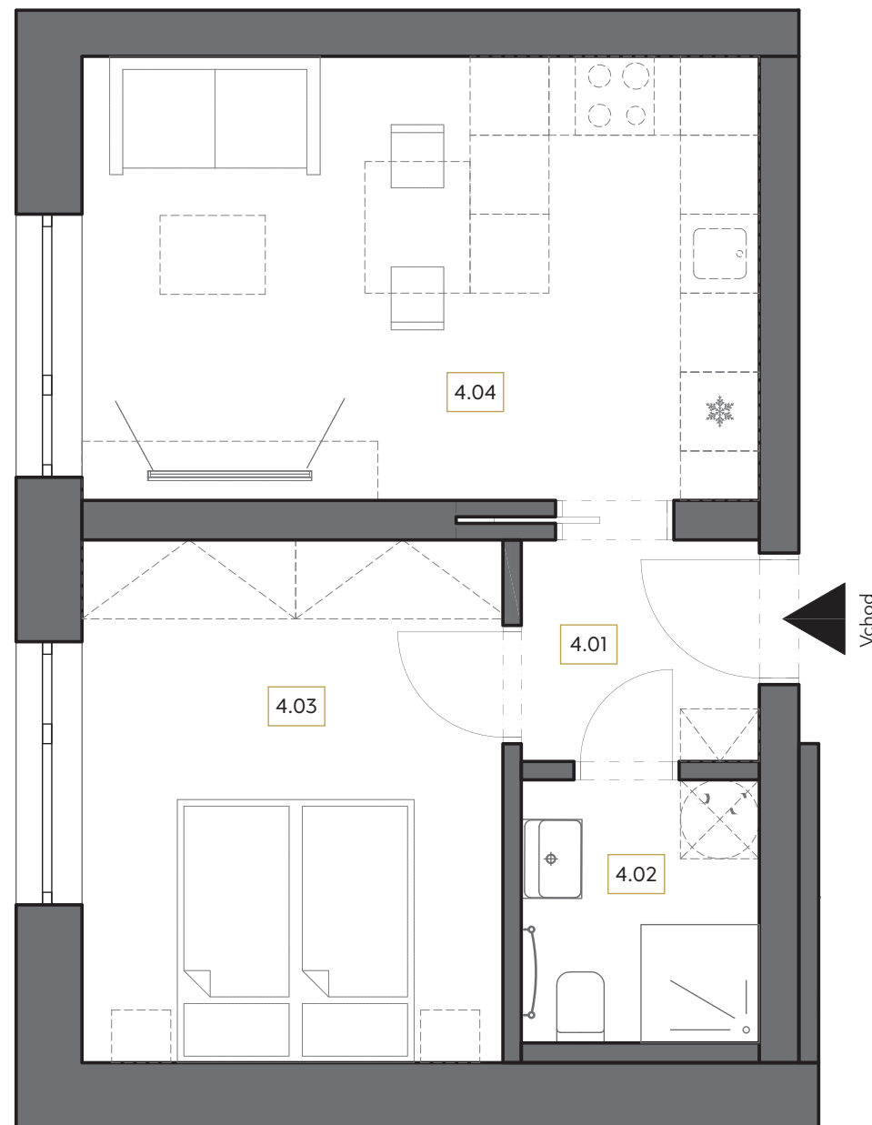
Půdorys bytu 4
